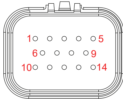
连接器背面
